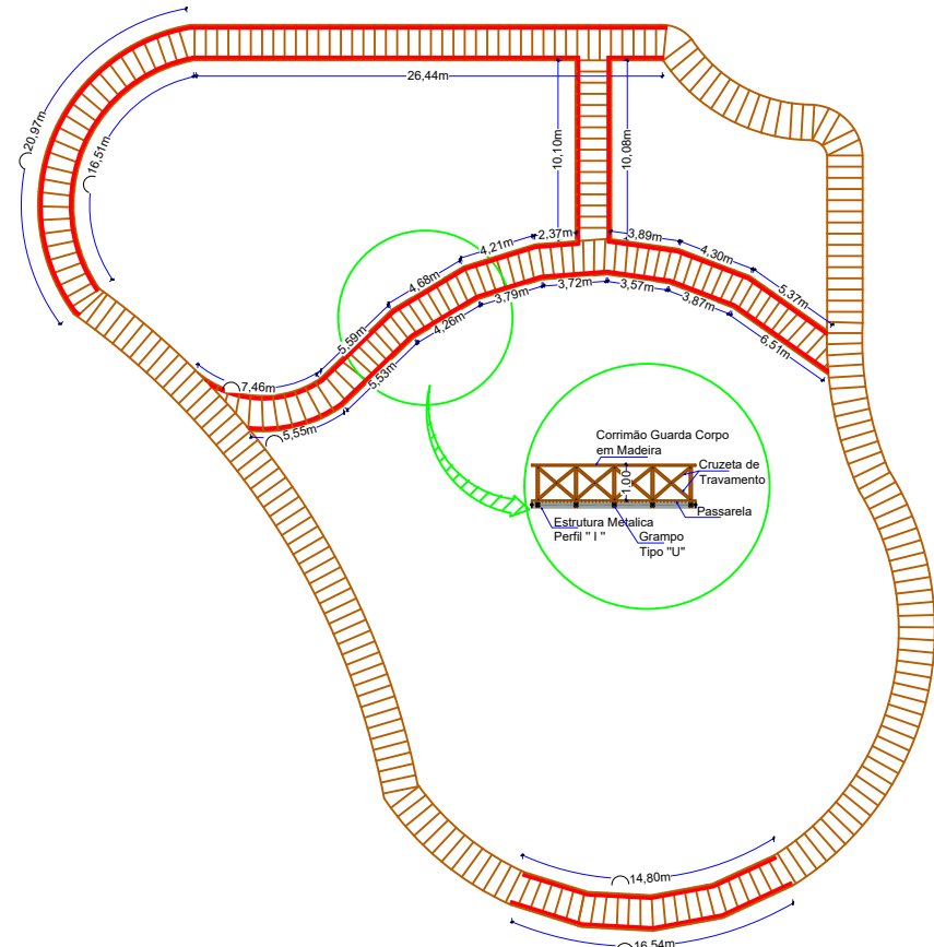
Locação do Guarda Corpo Esc: 1/200
