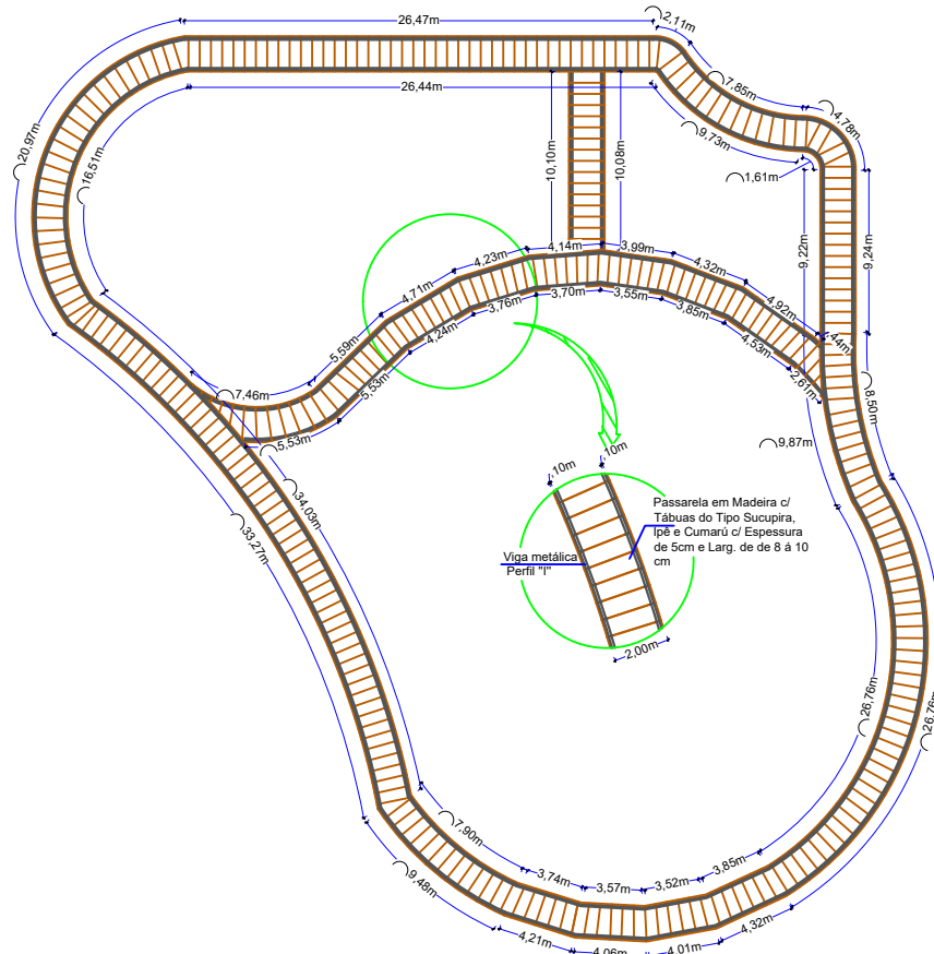
Planta Baixa - Passarela Esc: 1/200
