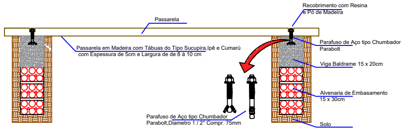
Det da fixação do Parafuso Parabolt na Madeira e na Viga de Concreto Esc: 1/10
